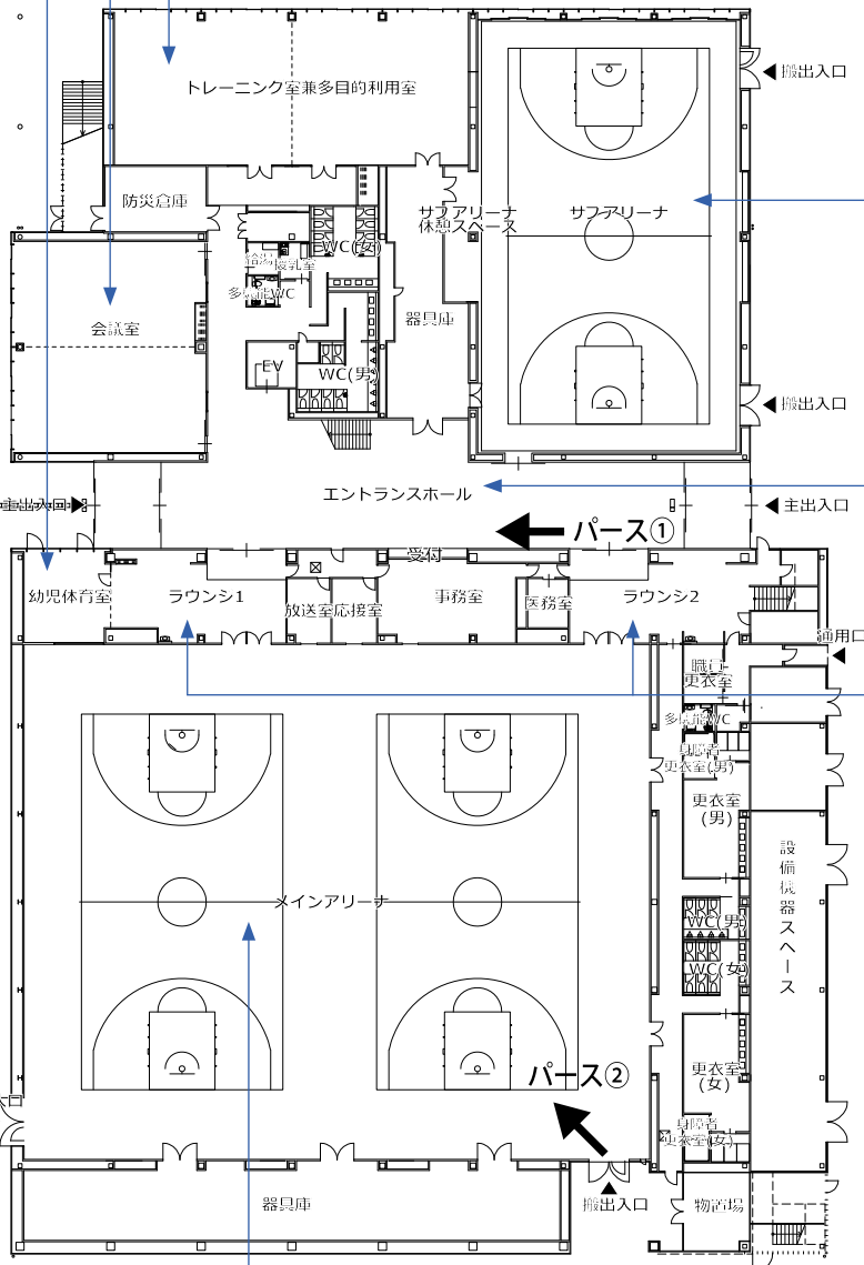
1階平面図
