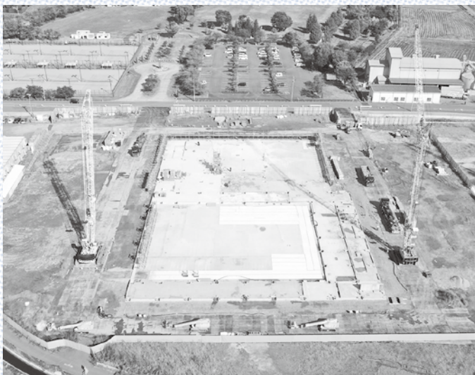
基礎および1階床コンクリート施工完了（南から北を望む）
