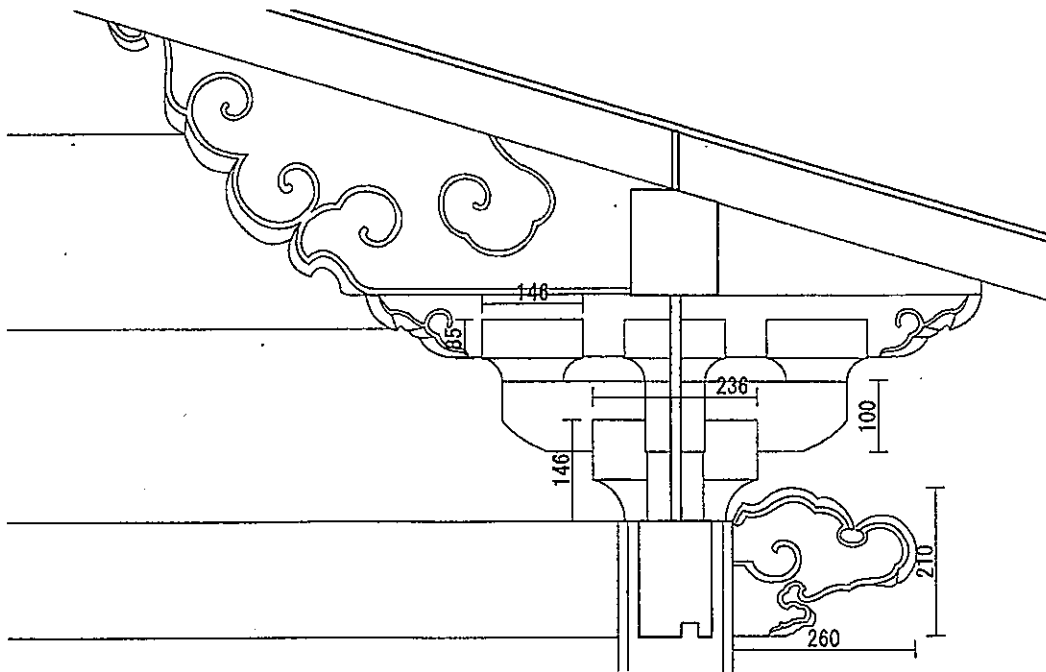
吉野神社本殿 断面詳細図 S=1/10
