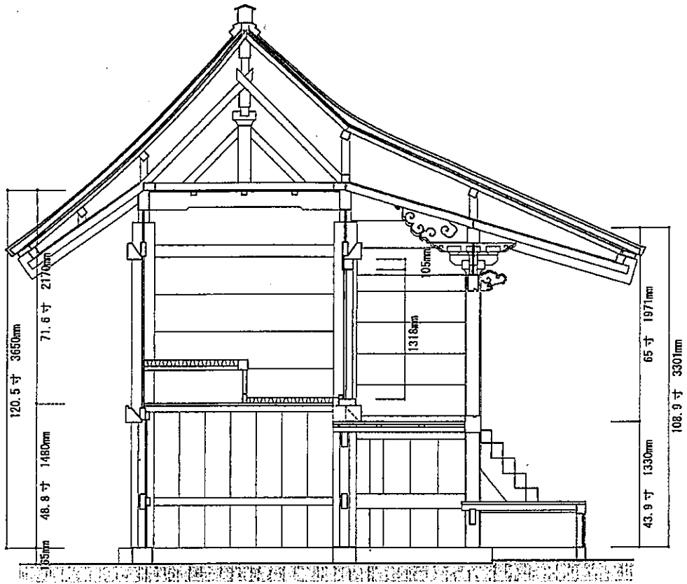
吉野神社本殿 断面図 S=1/50
