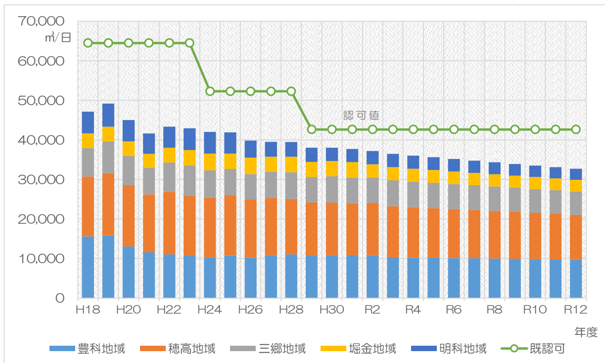
図 2-3 ■ 一日最大給水量の推移(安曇野市)
