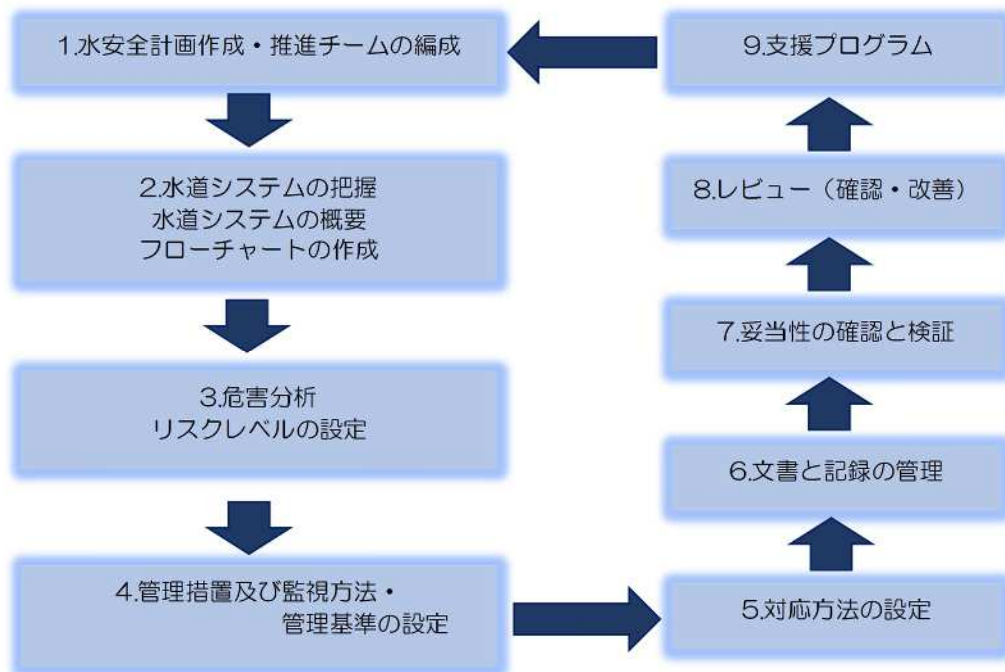
図 4-2 ■ 水安全計画策定の手順
