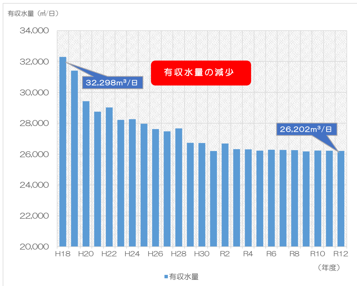
図 2-10 ■ 1日あたり有収水量の推移
