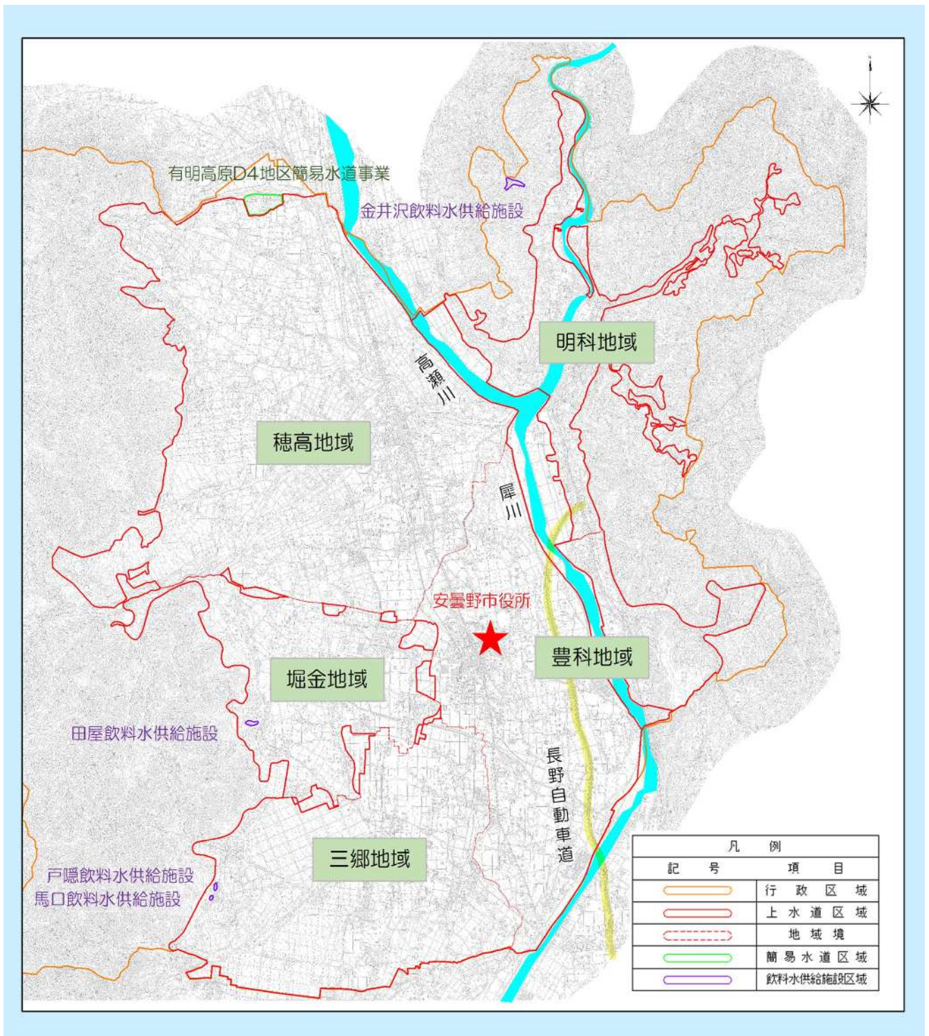
図 2-1 ■安曇野市水道施設位置図
