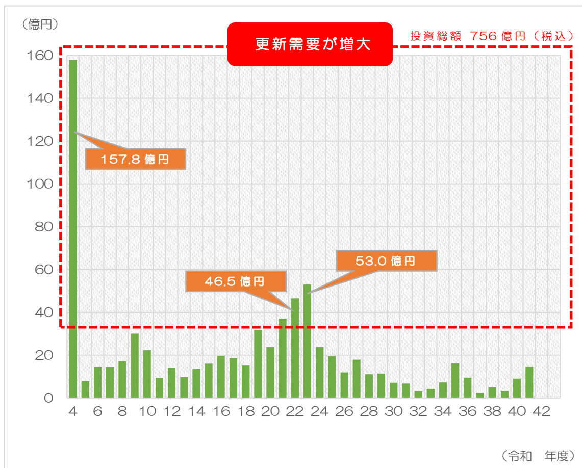
図 2-12 ■ 管路の更新需要 (法定耐用年数で更新)
