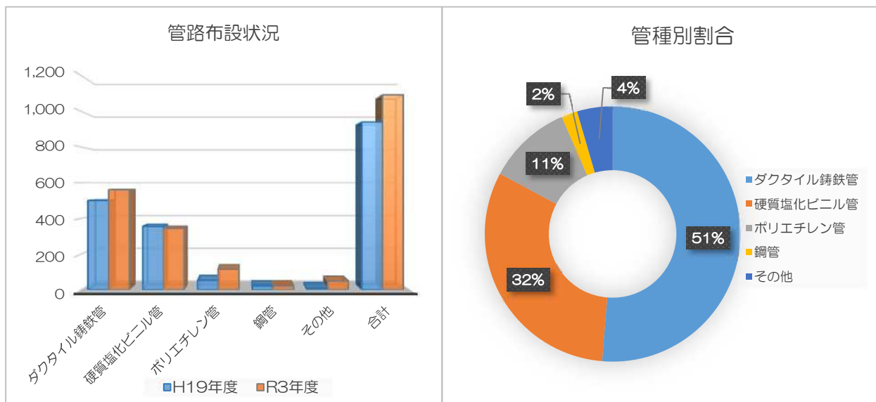
図 2-4 ■ 管路布設状況 (R3 年度末)
