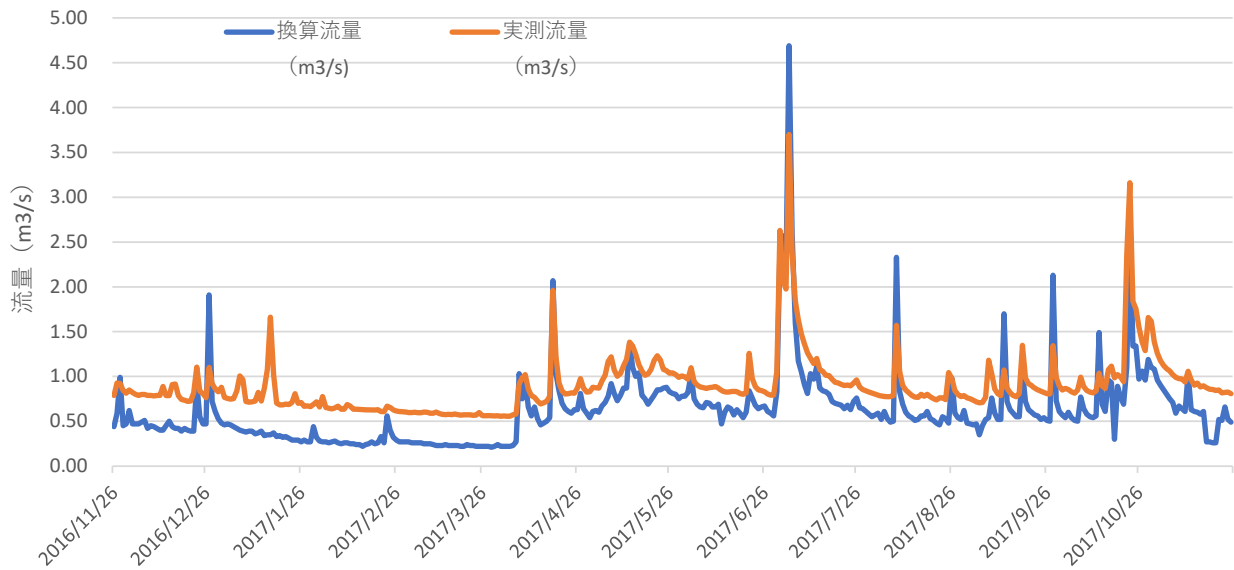
観測期間各日における日平均流量の比較（2016年11月～2017年11月）
