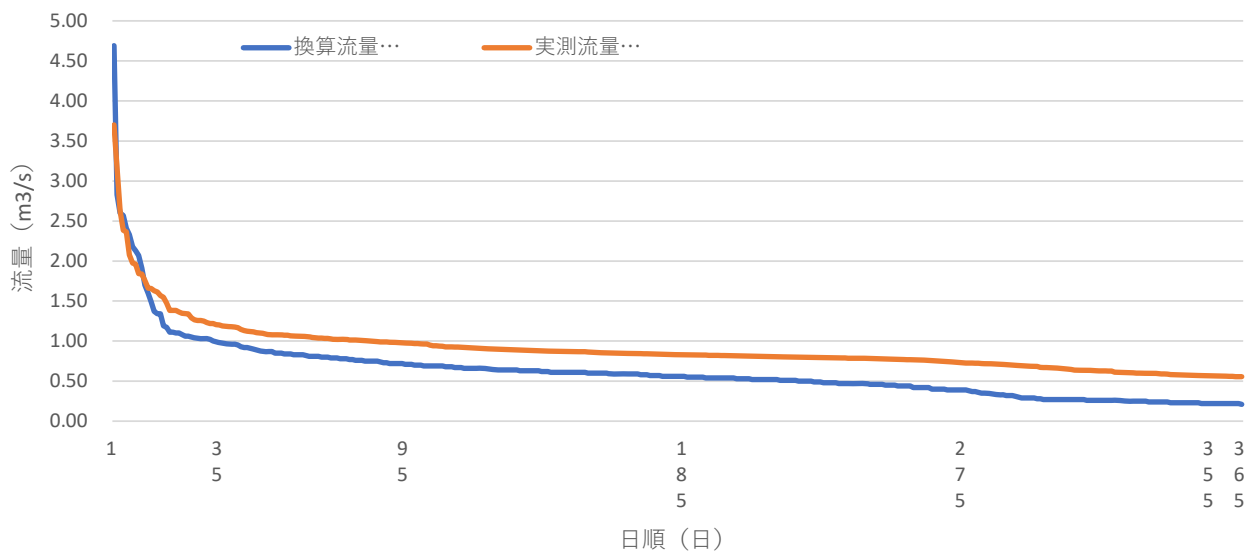
観測期間における流況曲線の比較（2016年11月～2017年11月）
