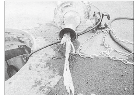
モップを巻き込み停止したポンプ （分解して除去しました）
