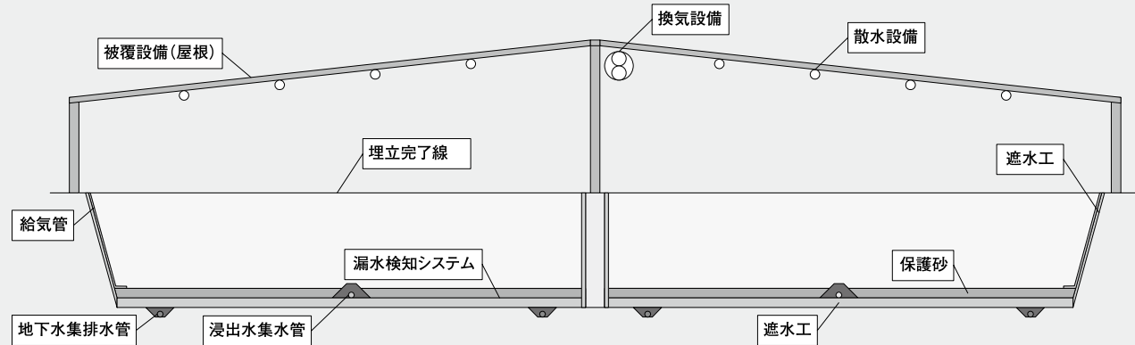
被覆型処分場の断面イメージ
