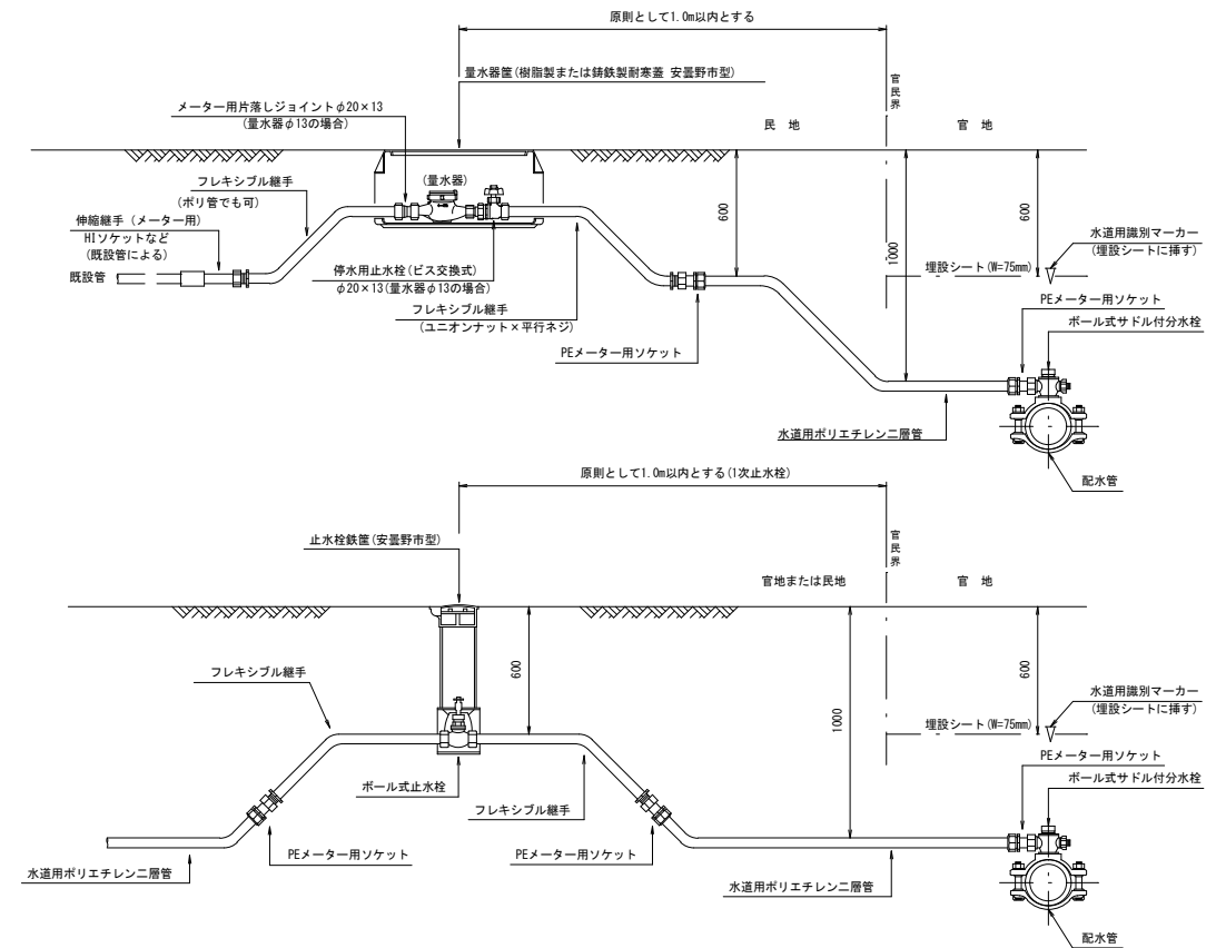
土工断面図
