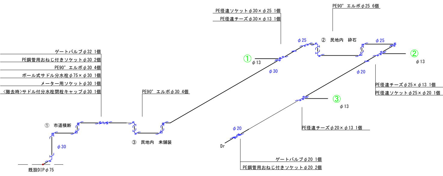
仮設配管標準土工断面図
