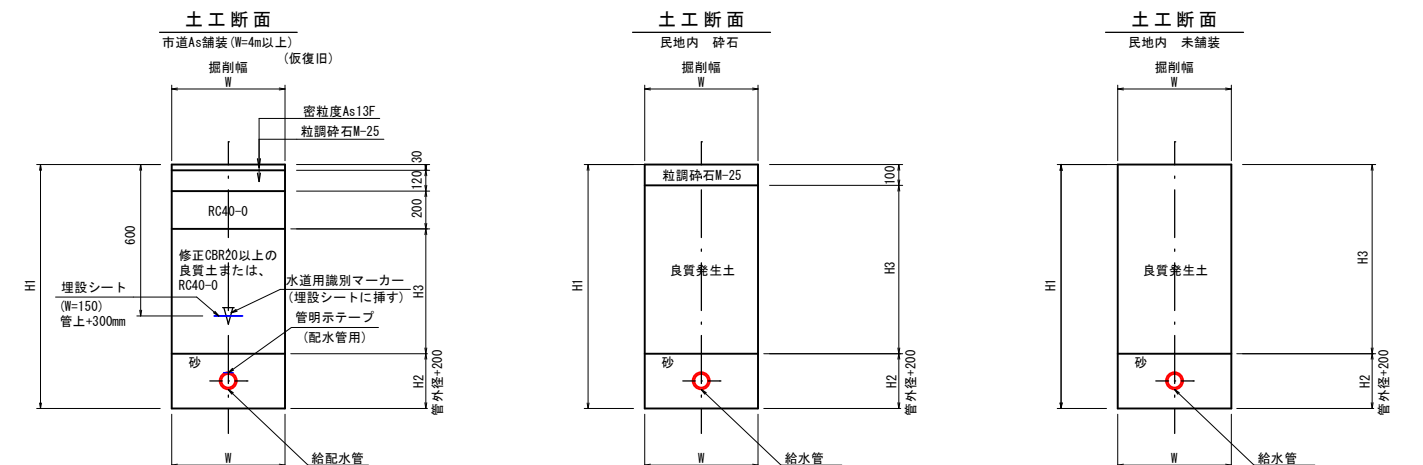
土工断面図
