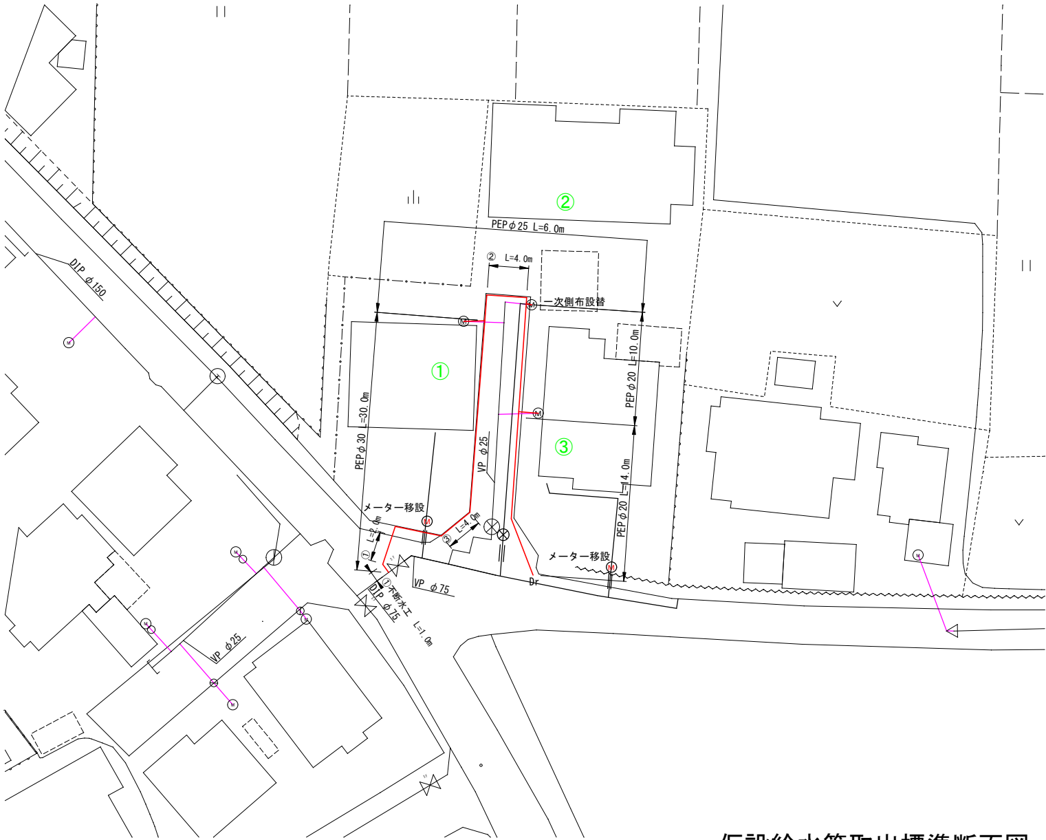
仮設給水管取出標準断面図
