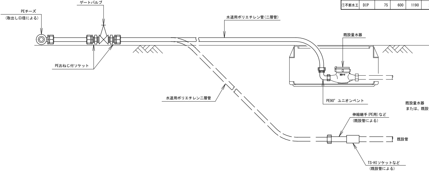
仮設給水管取出標準断面図
