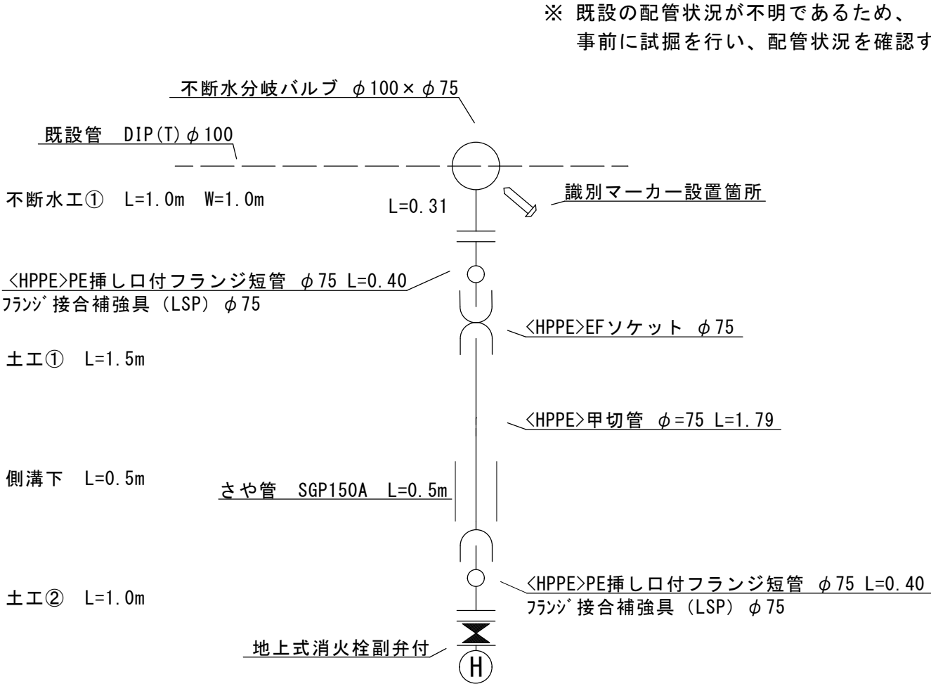
配管図
