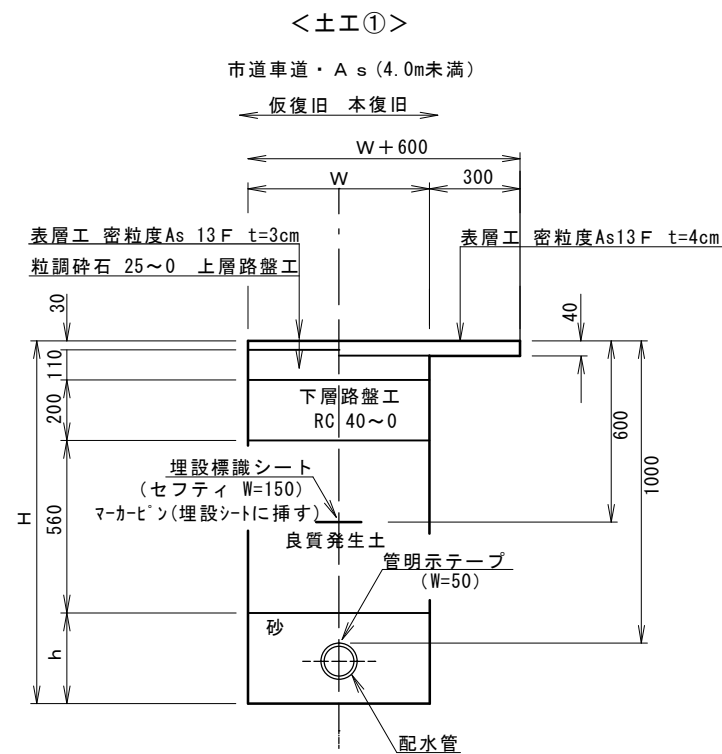
土工断面図
