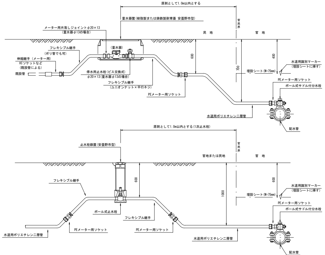
土工断面図
