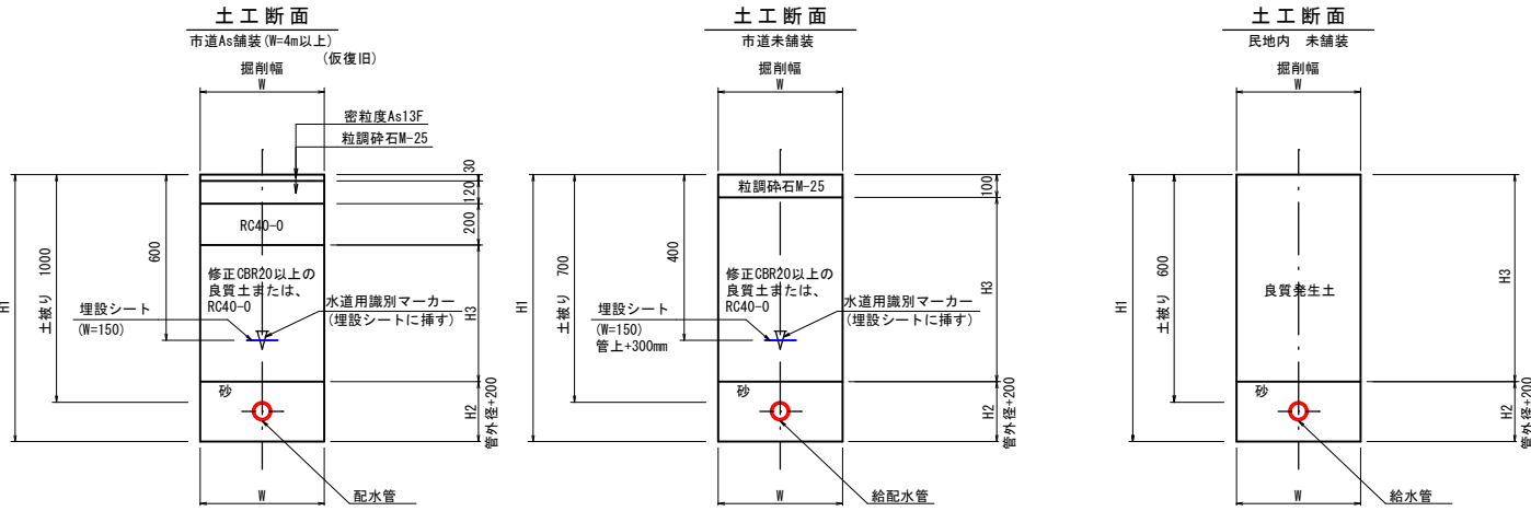
土工断面図
