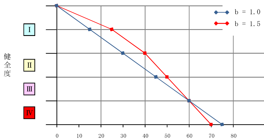
図3 劣化曲線の例
