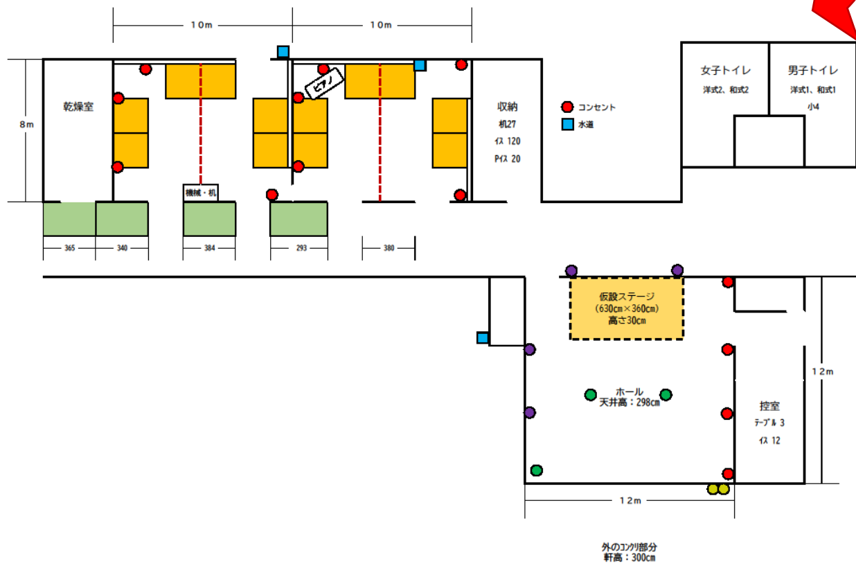
へいめんず うえ み へや はいち 平面図（上から見た部屋の配置など）
