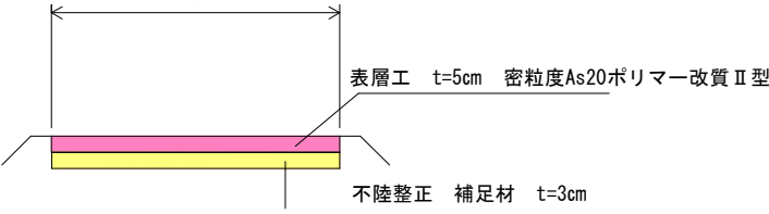
標準断面図(取付け舗装)
