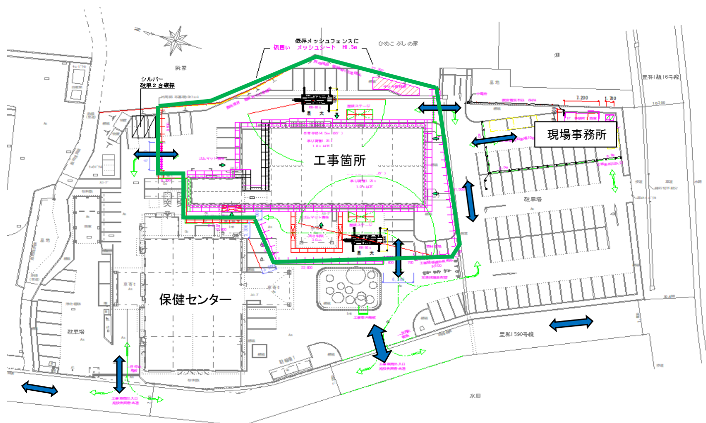
現場配置図（略図）
