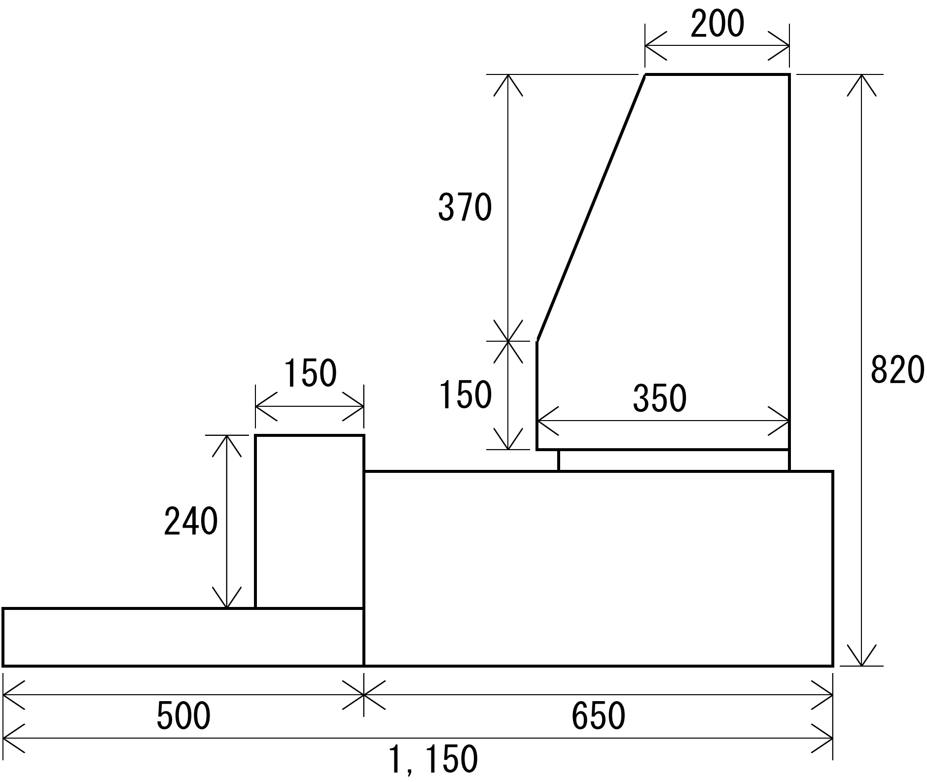
側面図
