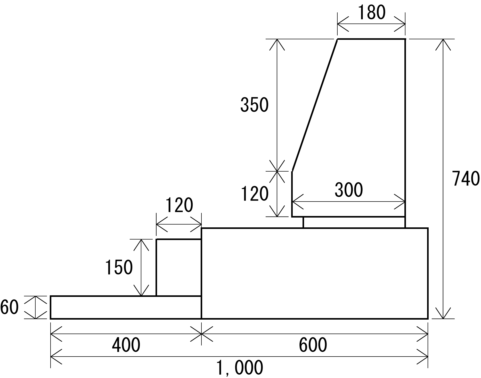
側面図
