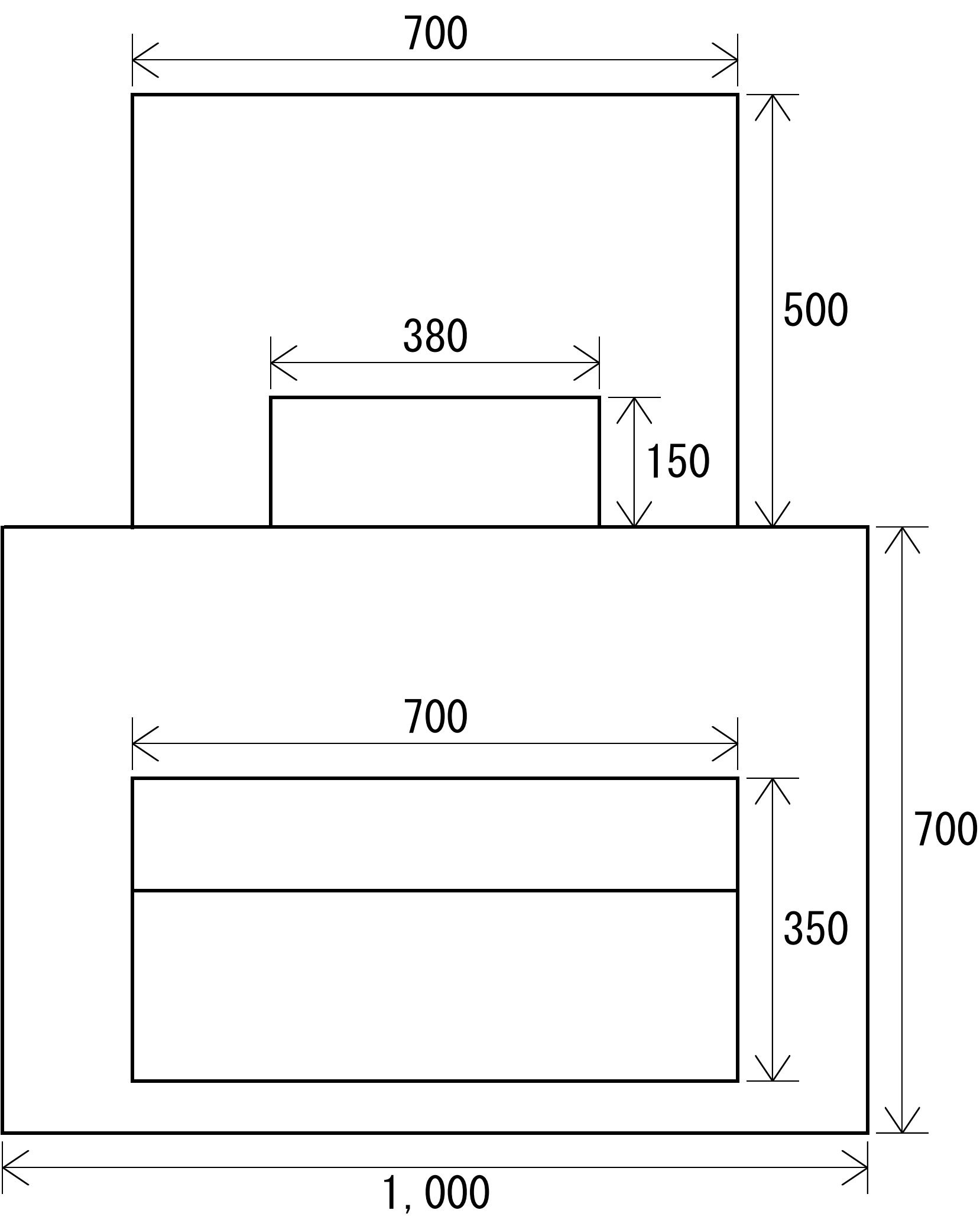
平面図
