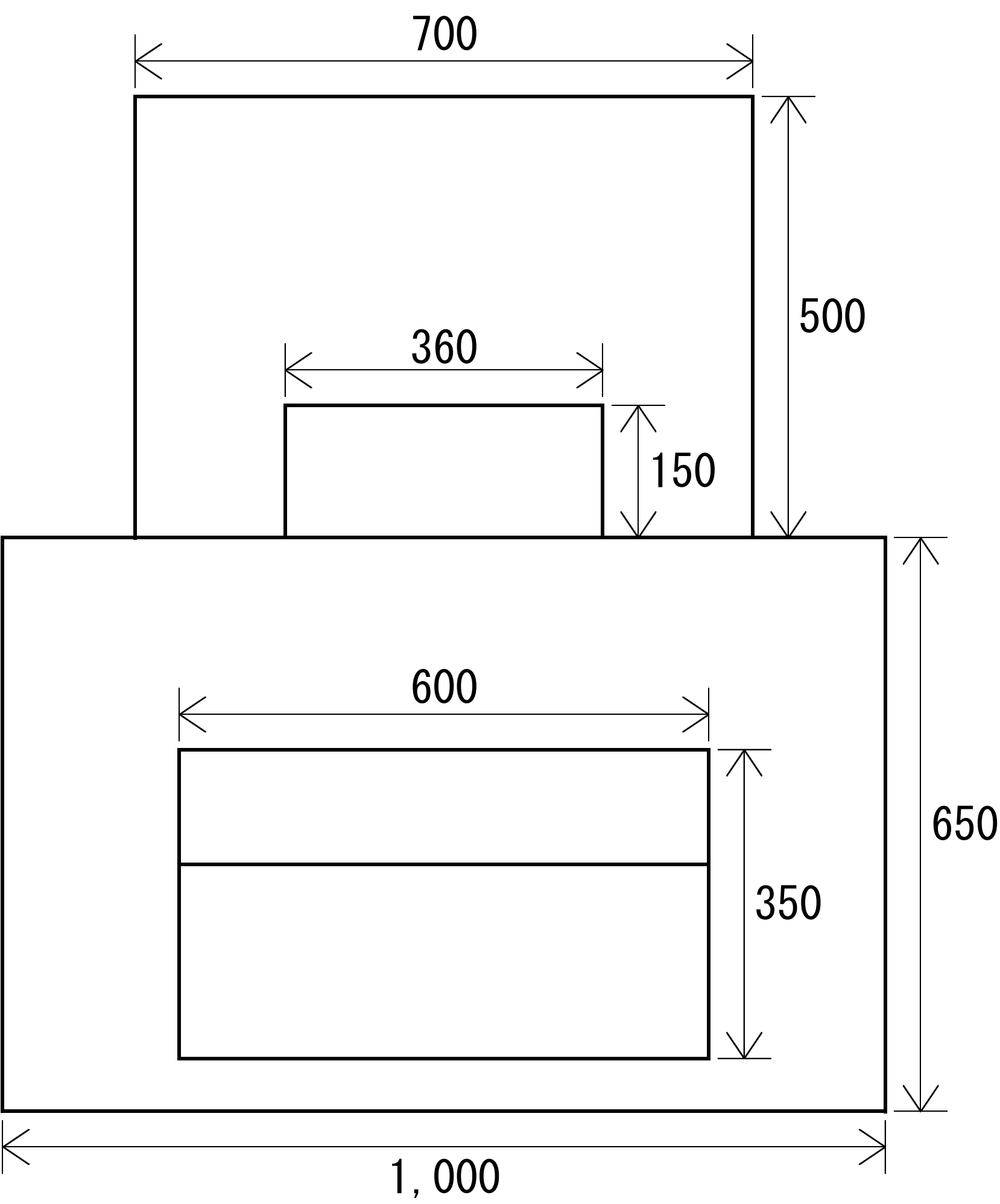
平面図
