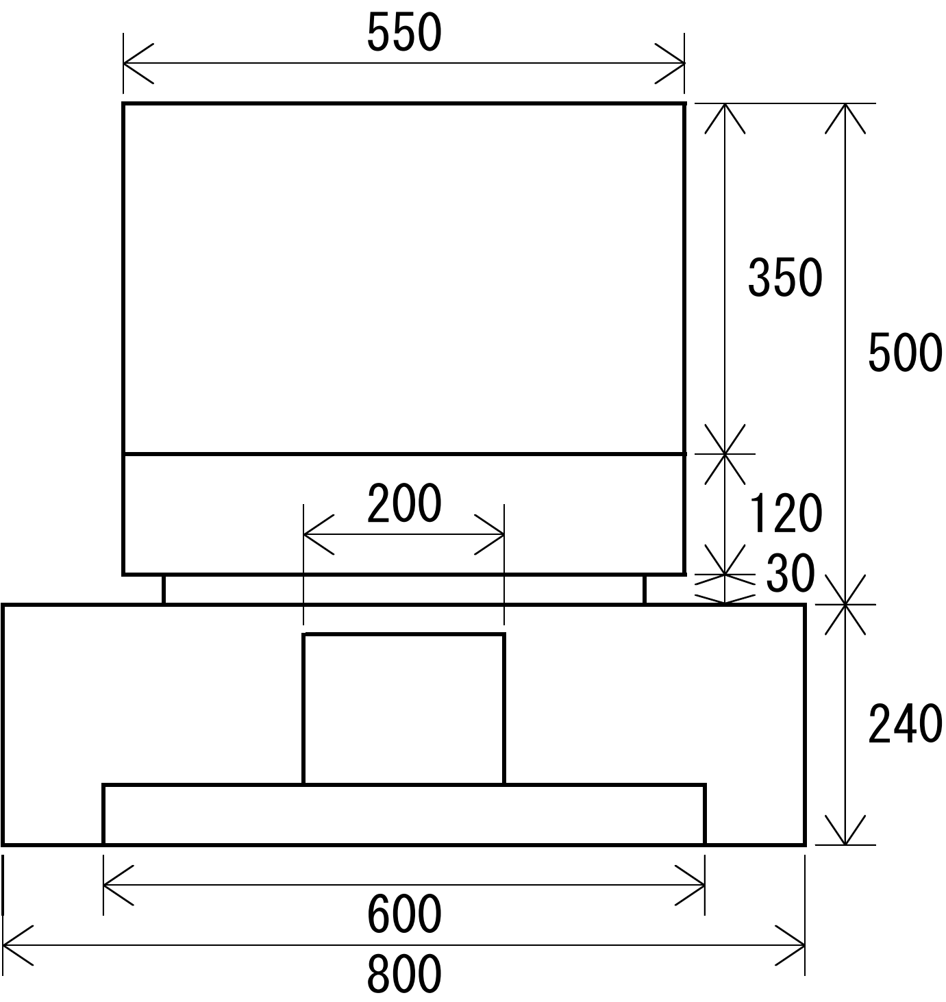
正面図
