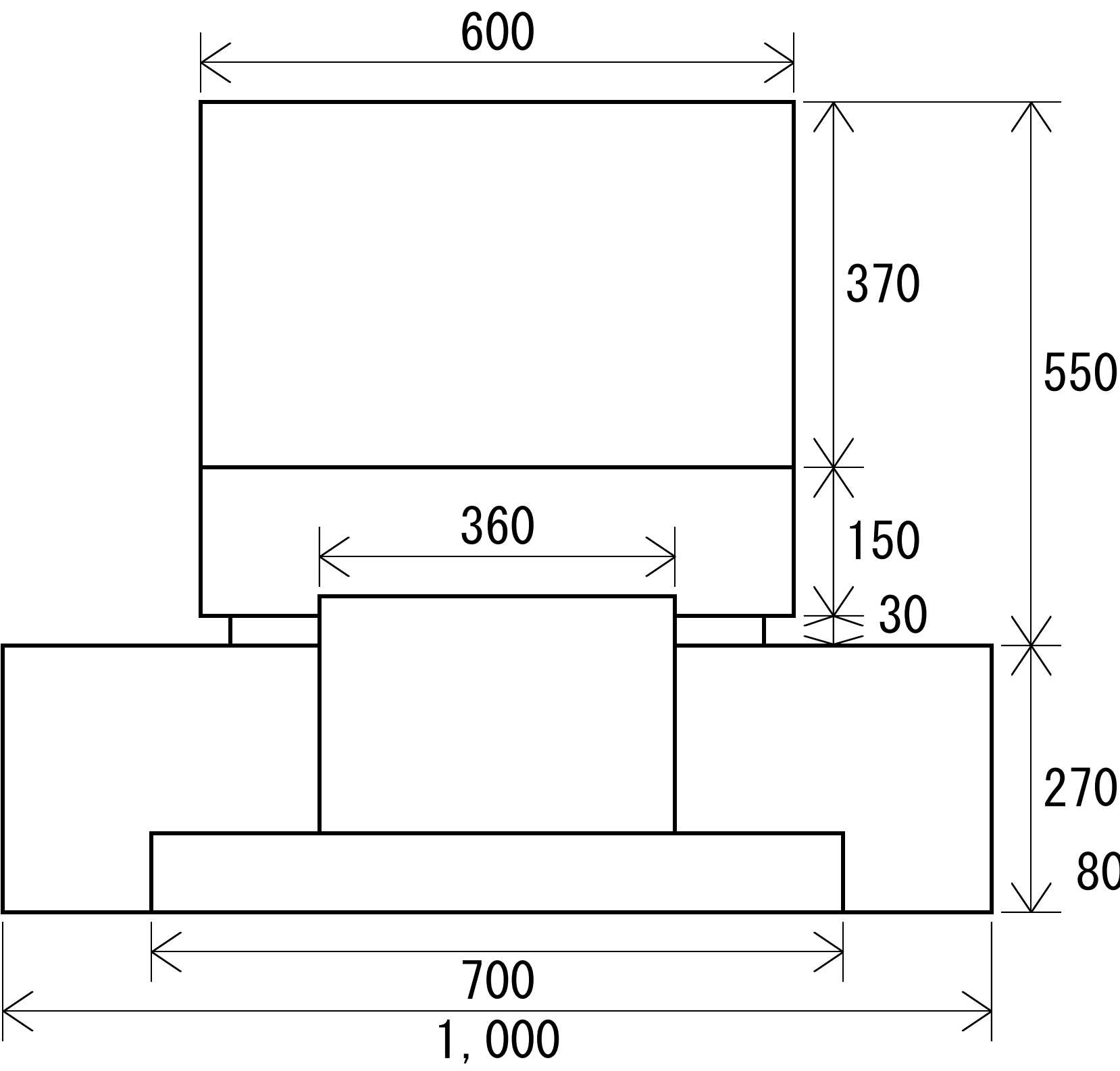
正面図
