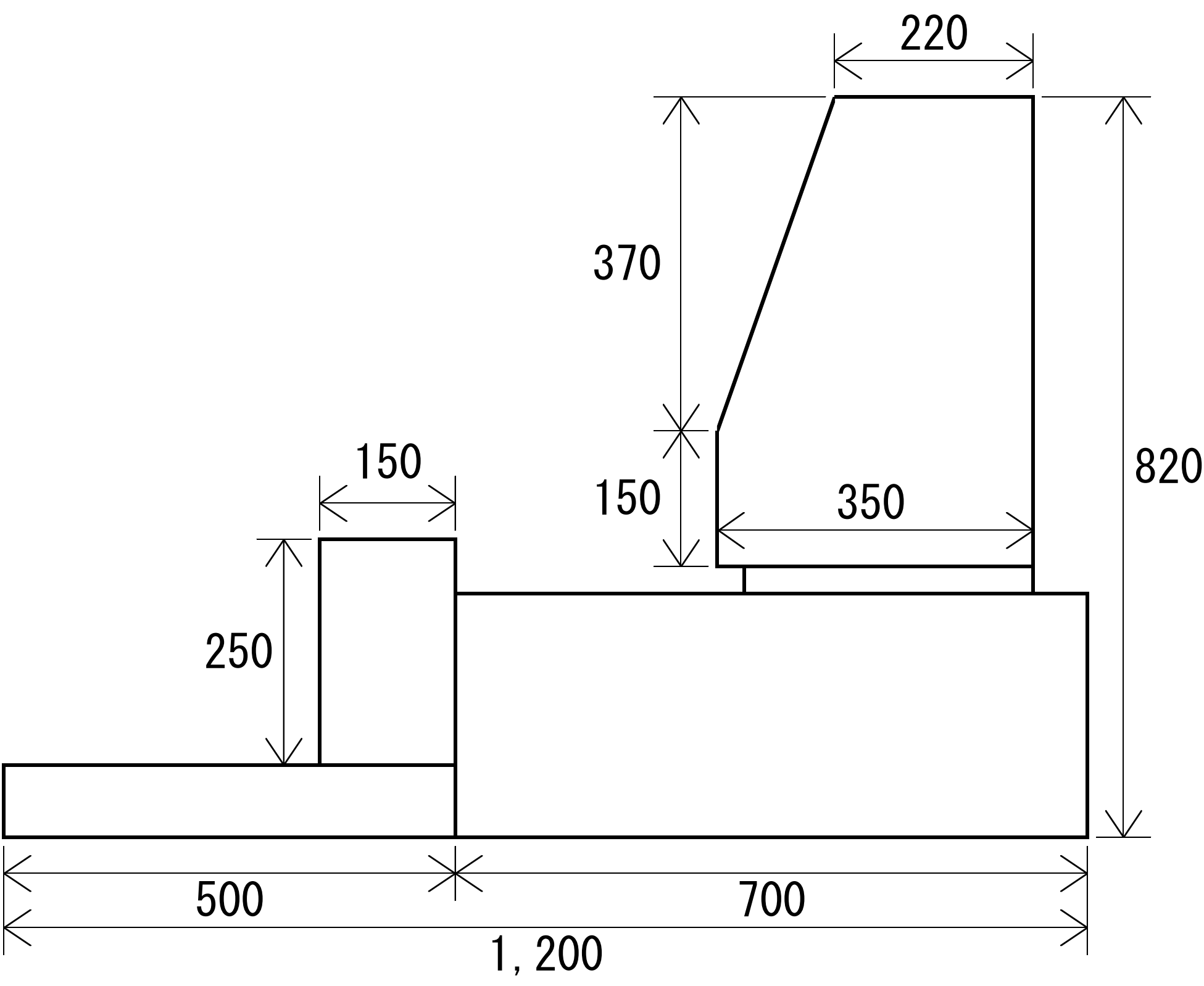
側面図
