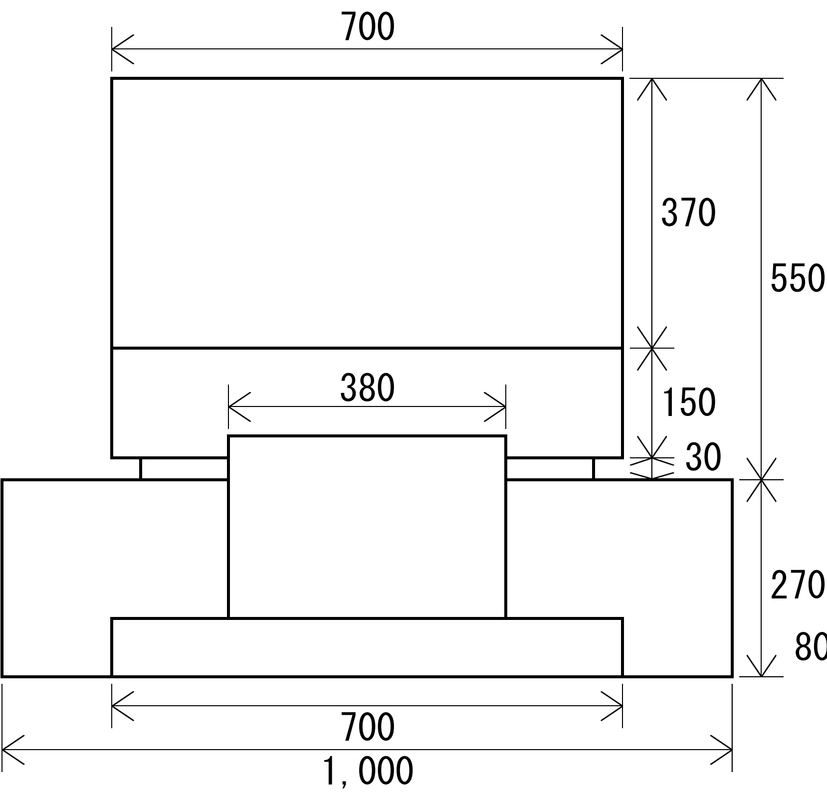
正面図
