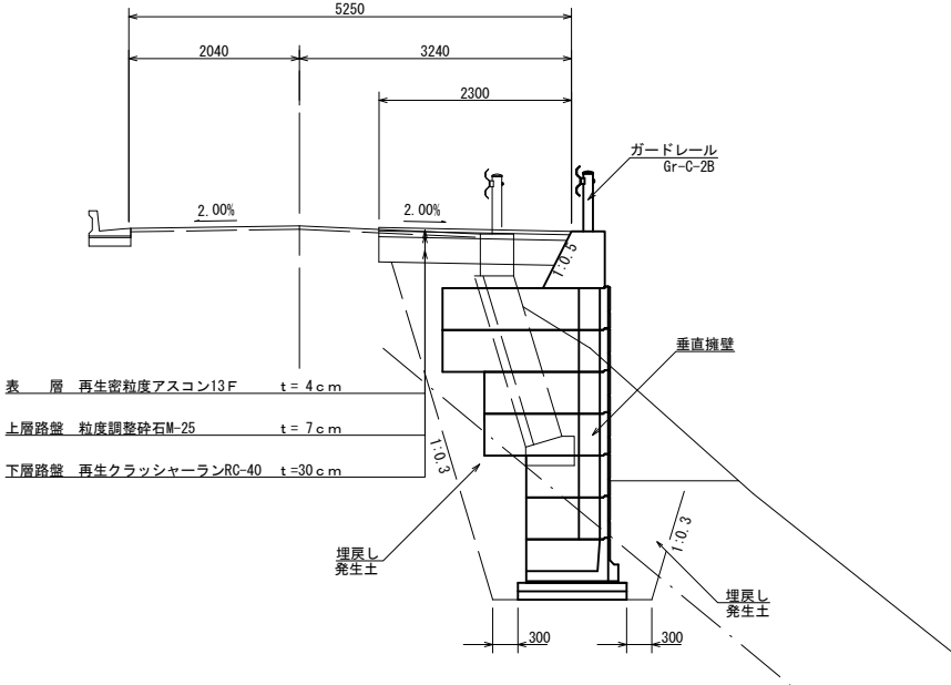
標準横断面図 S=1:50 EC. 1
