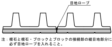
目地ロープ・詳細図
