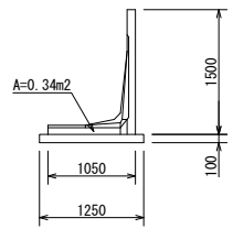
L型擁壁
