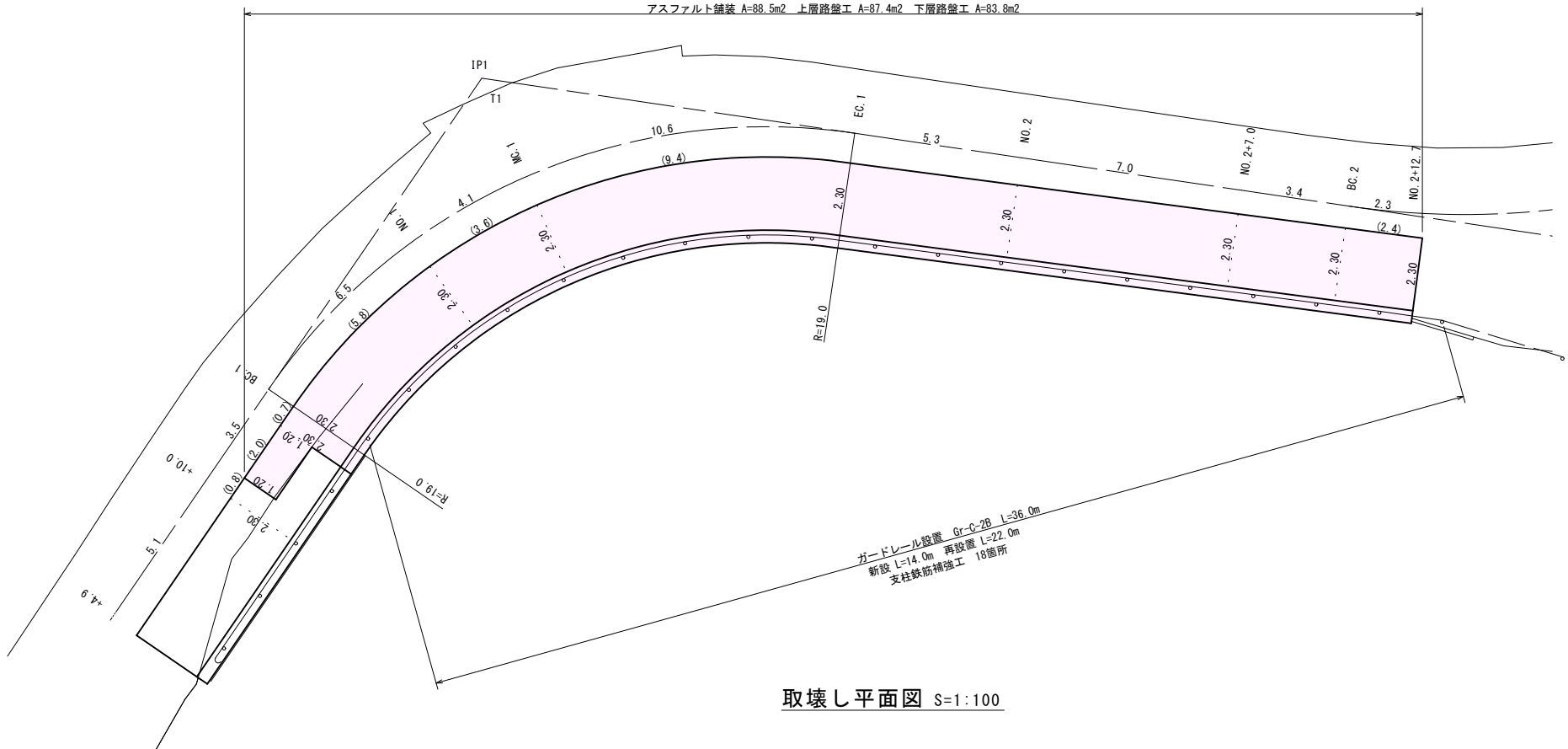
アスファルト舗装平面図 S=1:100
