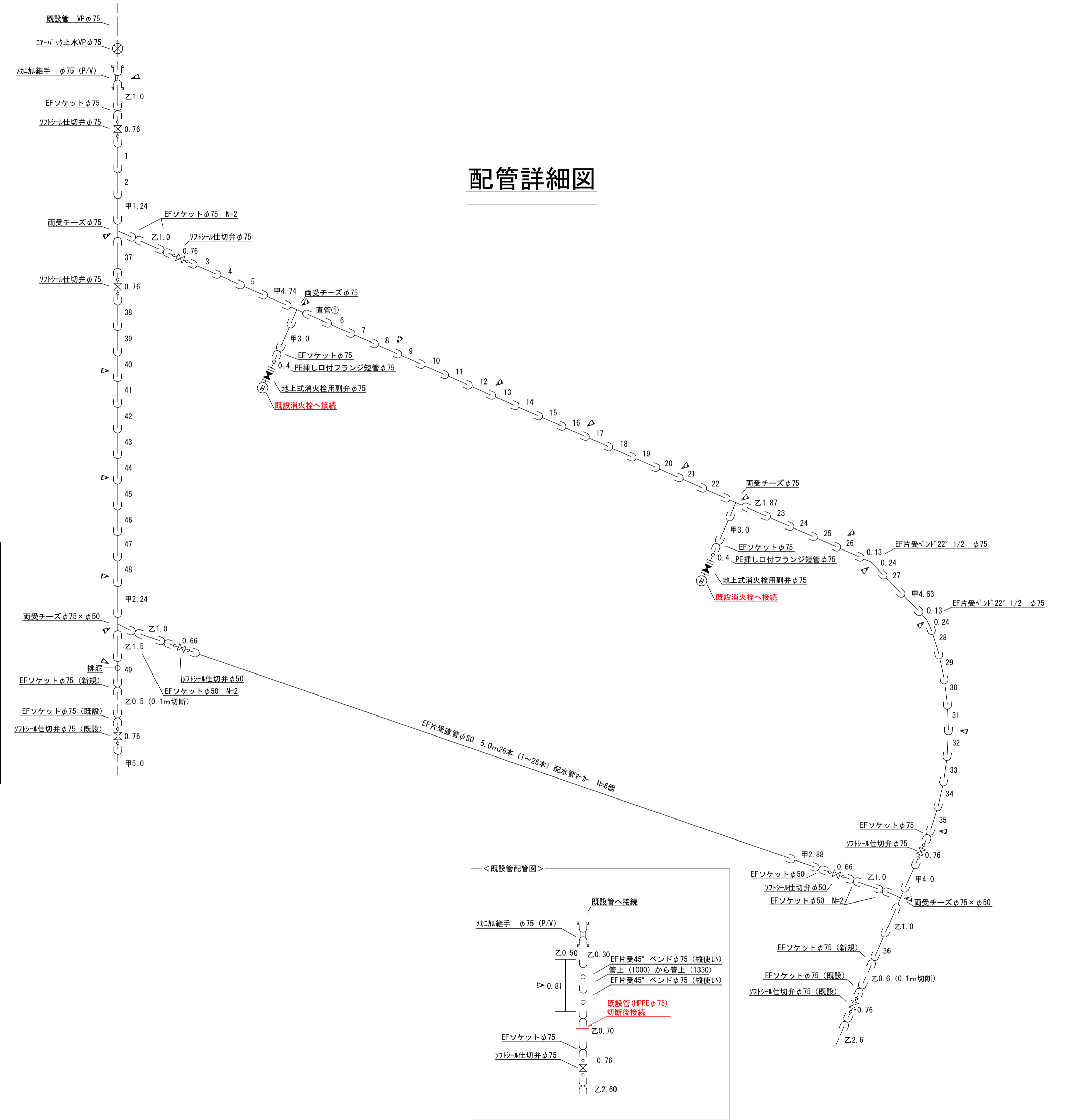
実施図
