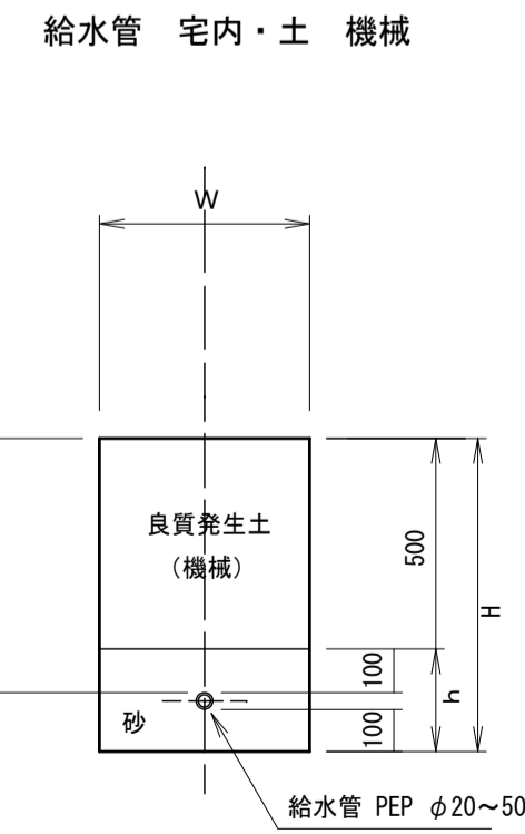
土工断面
