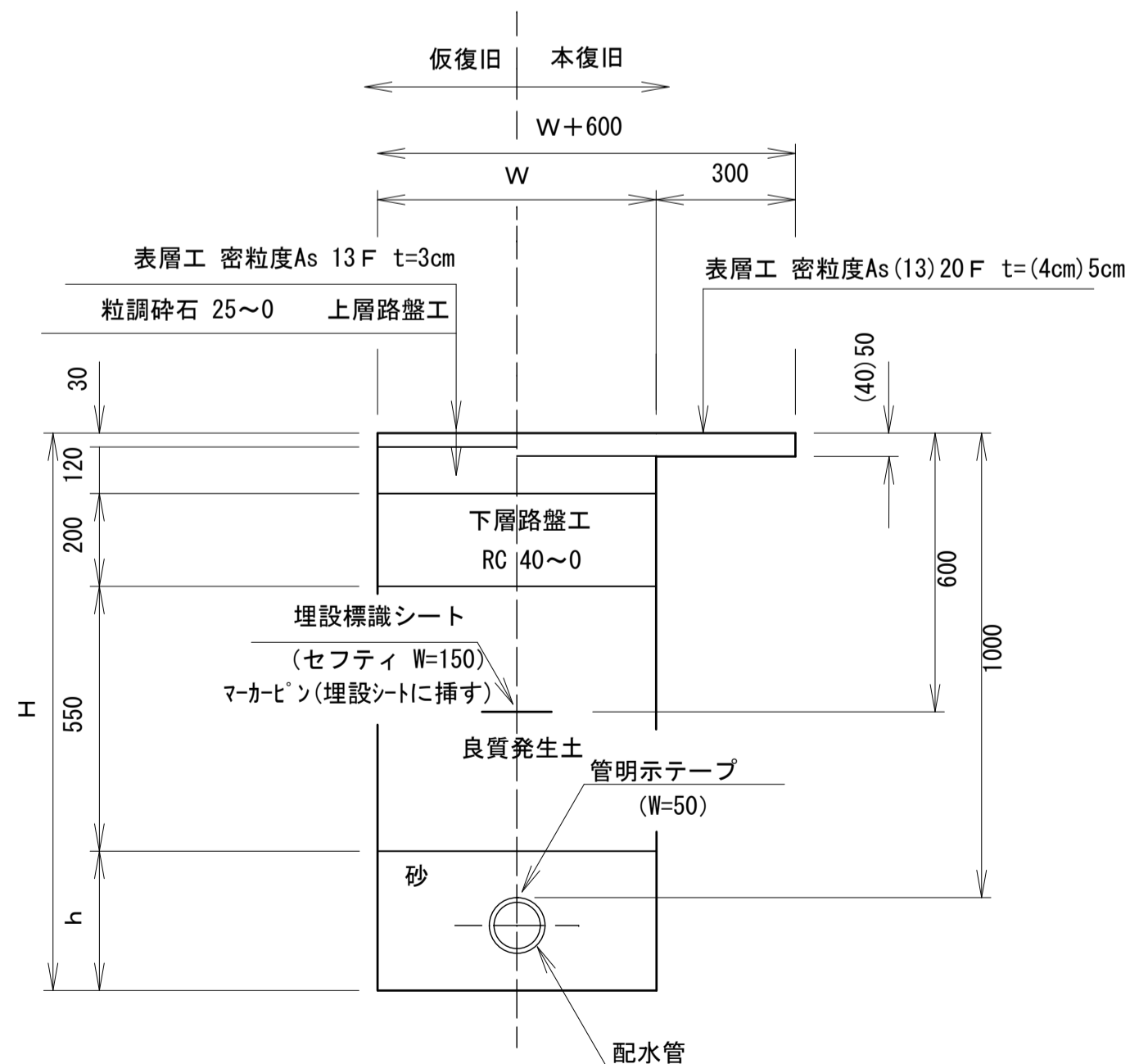
給・配水管公道内土工
