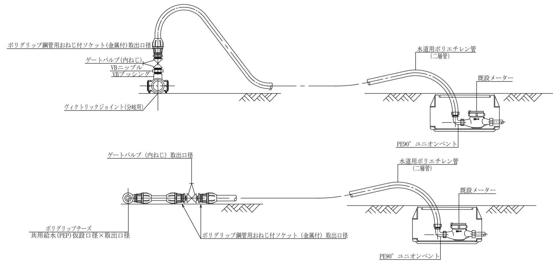
仮給水管標準断面図
