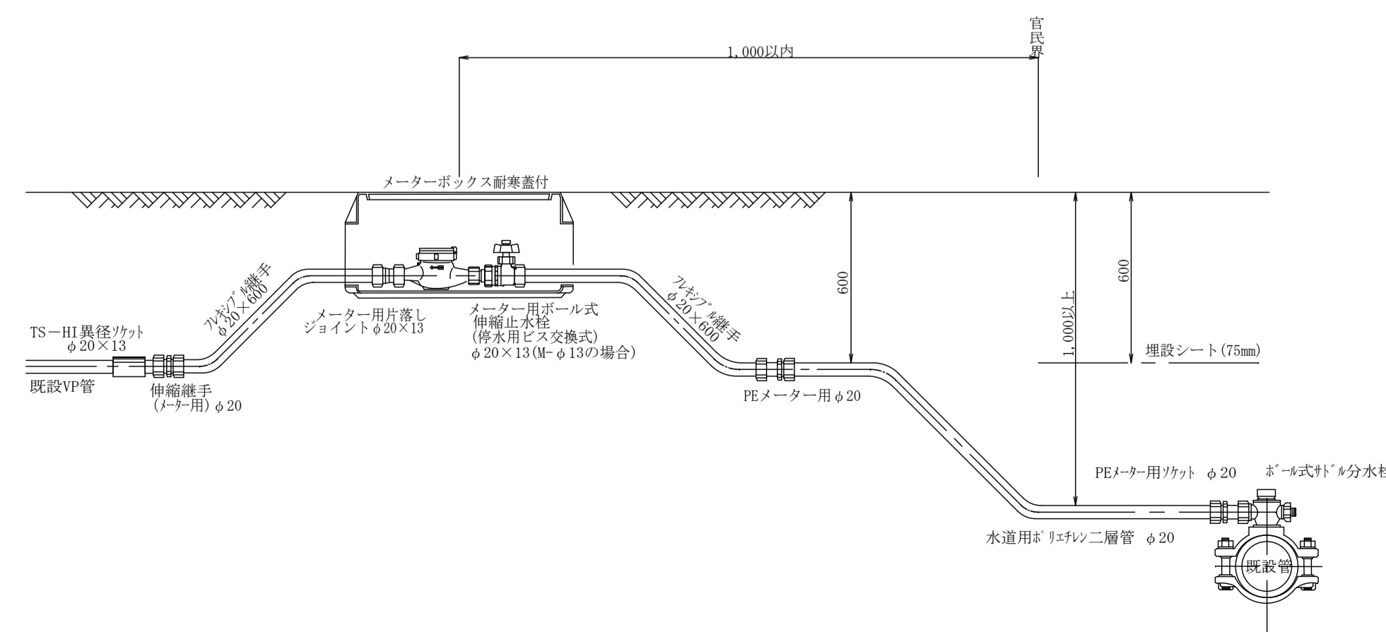
給水管標準断面図
