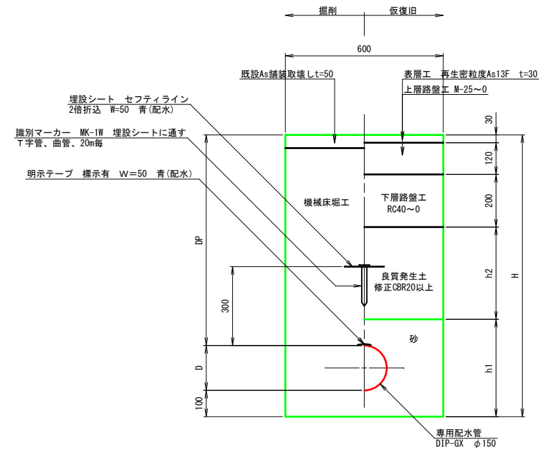
土工断面 1 市道車道・As（舗装幅員4m以上）仮復旧
