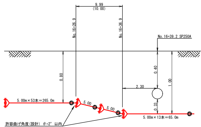
A-A横断面図
