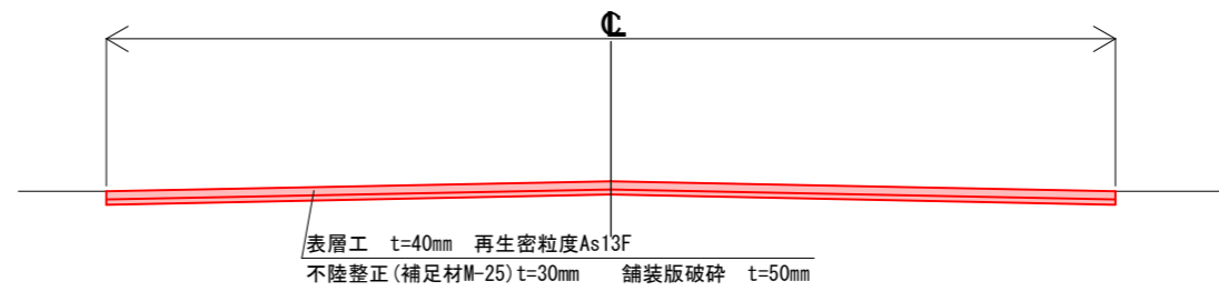
標準断面図
