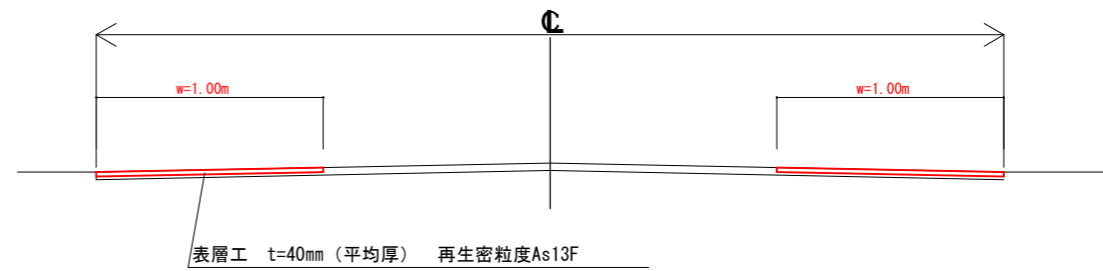
標準断面図
