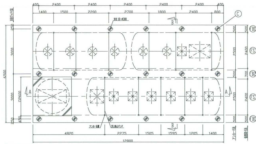
基礎伏図 S=1/50
