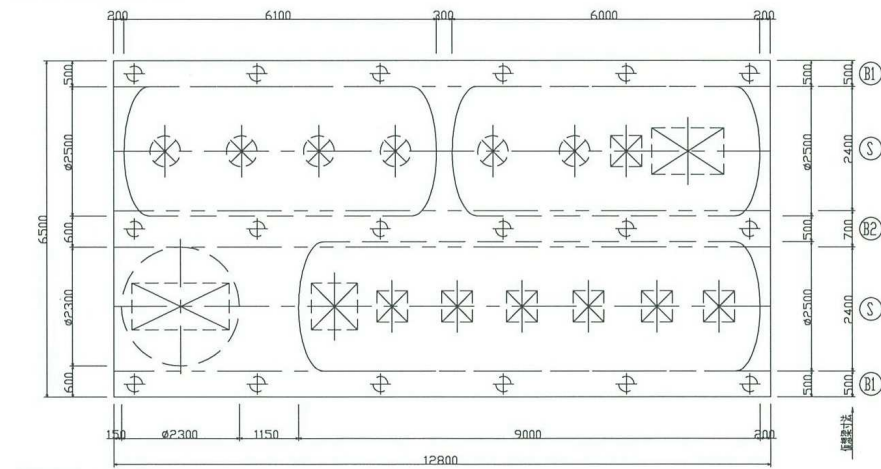
床伏図 S=1/50
