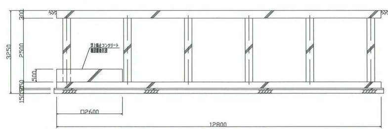
A-A 断面図 S=1/50
