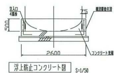
浮上防止コンクリート図 S=1/50
