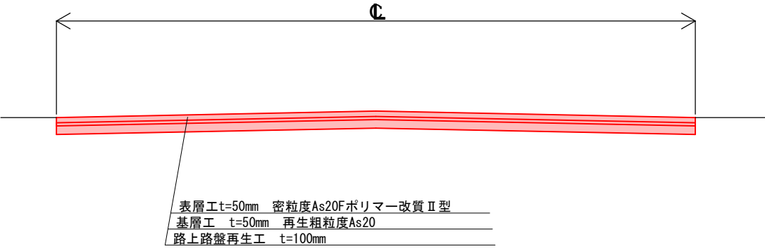
標準断面図
