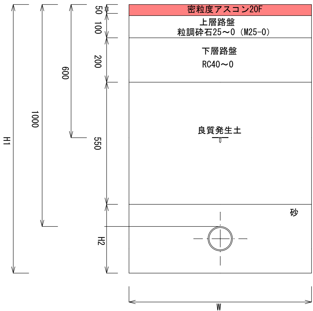
市道 復旧標準図
