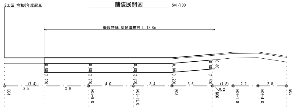
舗装展開図 S=1/100
