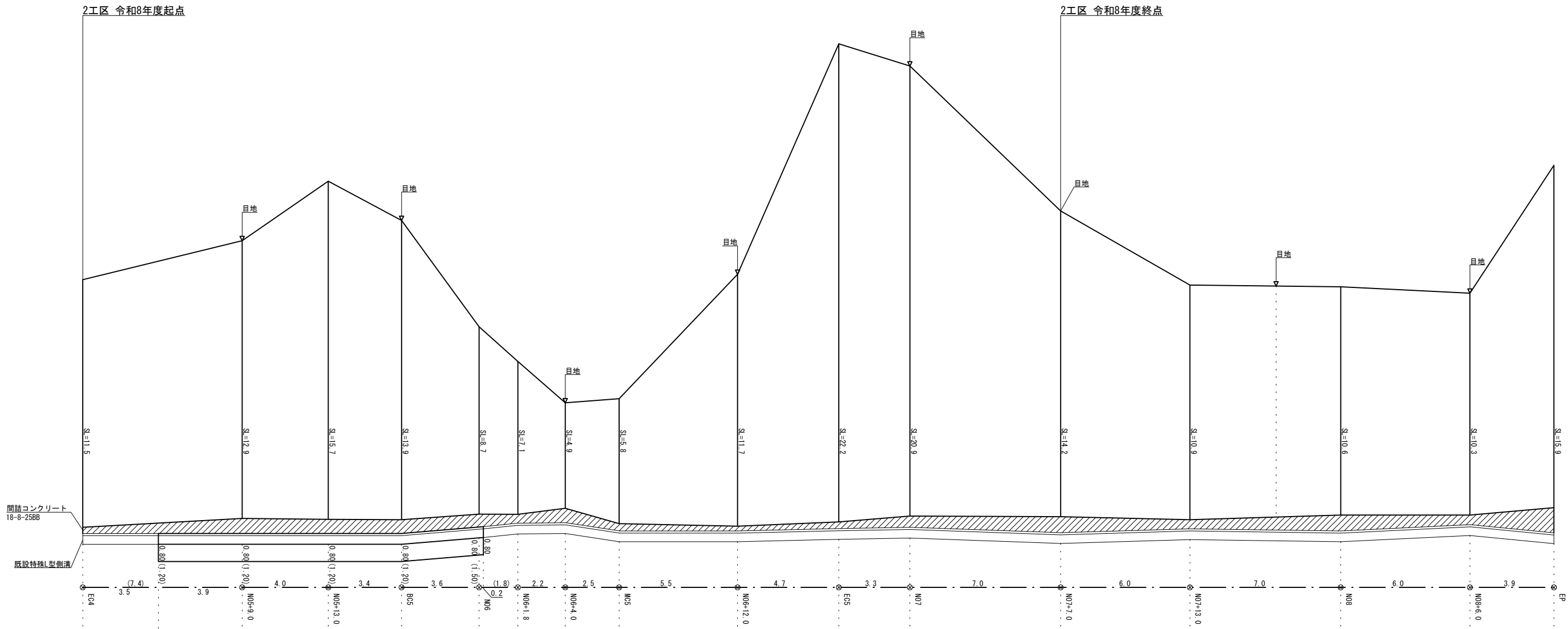
コンクリート吹付法面展開図 S=1/100
