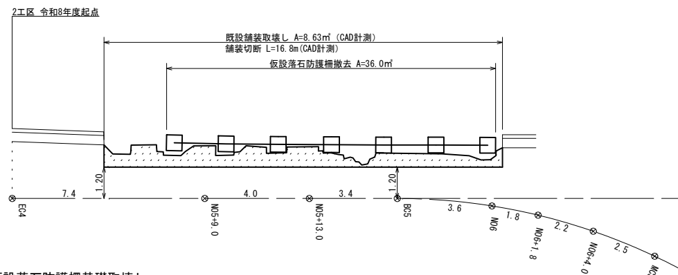
仮設落石防護柵基礎取壊し S=1/100
