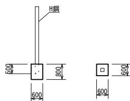
仮設落石防護柵基礎取壊し S=1/100
