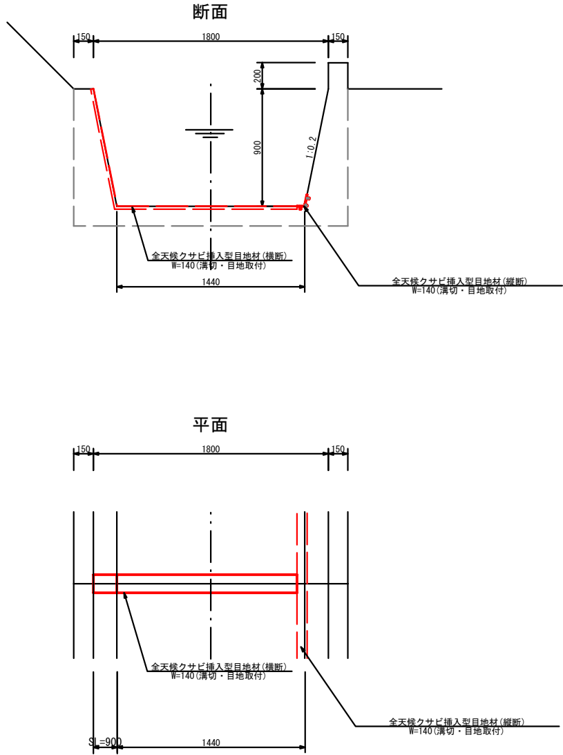
標準断面図 S=1/20
