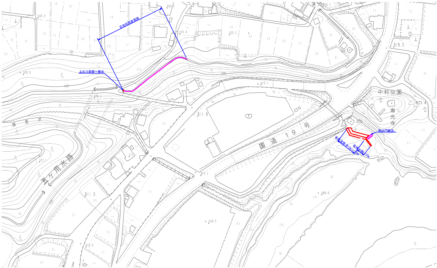
仮設計画図 S=1/1,000
