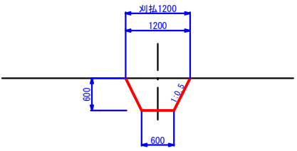
仮排水路 S=1/50
