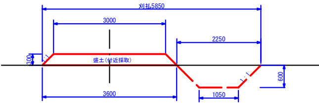
仮設道路 S=1/50
