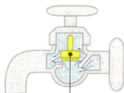
節水コマ
