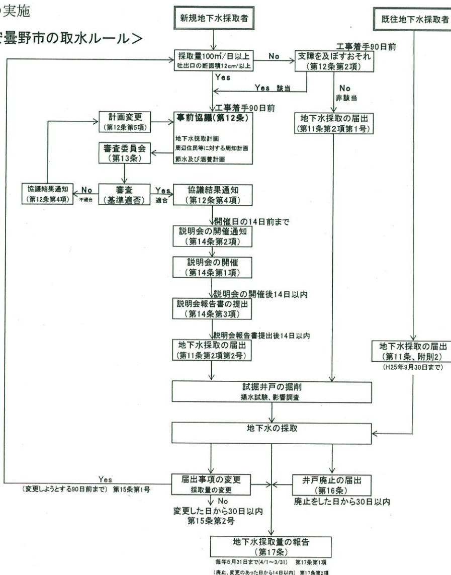
図 2.47 安曇野市の取水ルールフロー
