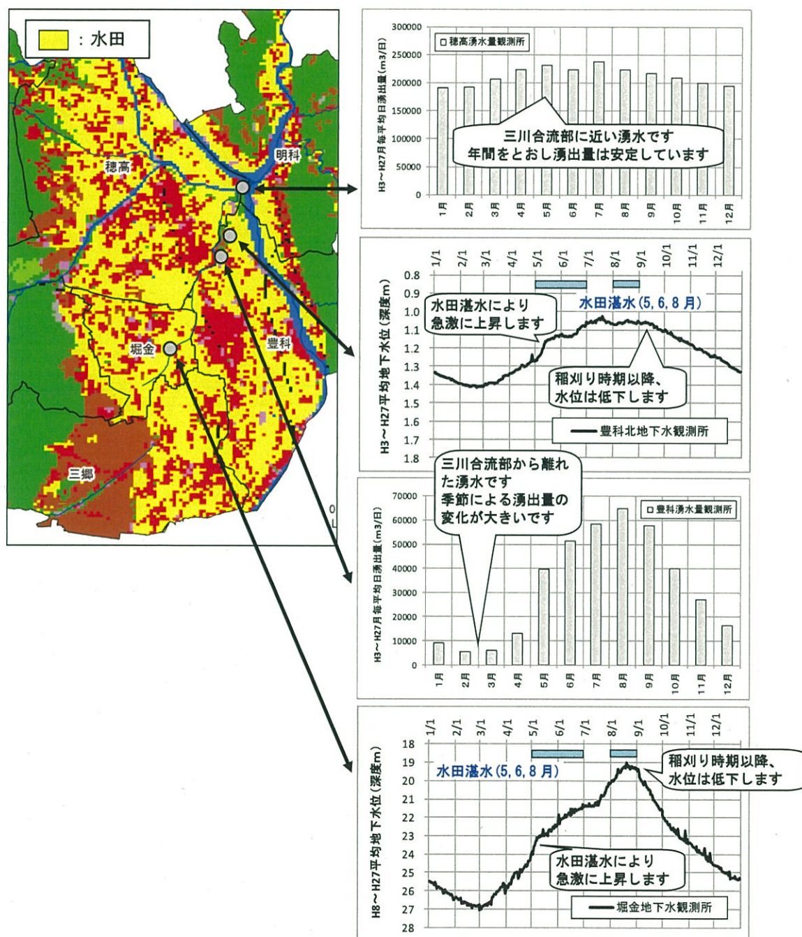
図 2.22 地下水位・湧出量の年間変化
